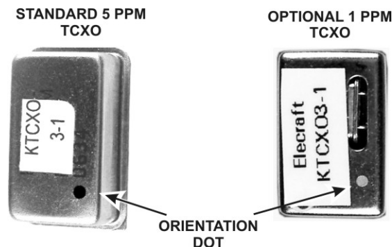
Figure 67. TCXO Modules.
